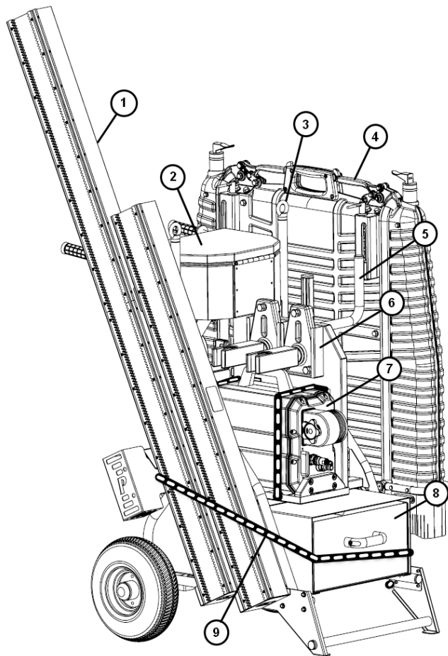
Carro de transporte cargado, parte delantera
